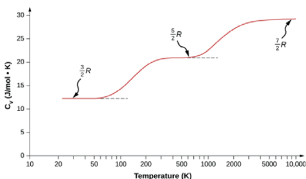
Fot. 3. Ciepło właściwe wodoru ( H_2 ) w funkcji temperatury (skala logarytmiczna) [8]. Ciepło właściwe gazów jest niezwykle proste koncepcyjnie: c_v dla gazów atomowych wynosi 3/2 R (trzy kierunki ruchu translacyjnego) a dla drobin dwuatomowych 5/2 R (dodatkowo dwa kierunki rotacji). Ale „przydziałem” energii rządzi mechanika kwantowa: jeśli temperatura jest zbyt niska, niemożliwe są rotacje; a w wysokich temperaturach drobina zaczyna drgać: pojawia się dodatkowe kT kwantu wzbudzenia wibracyjnego.
